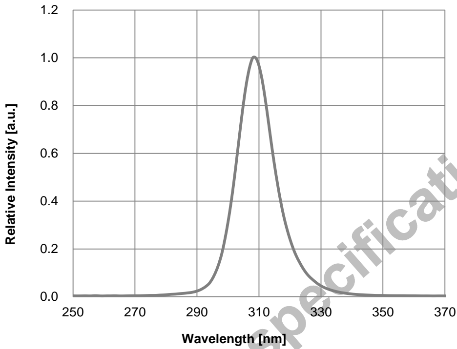
Fig 1. Spectrum, T_a=25^\circ\text{C} , I_f=100\text{mA}
